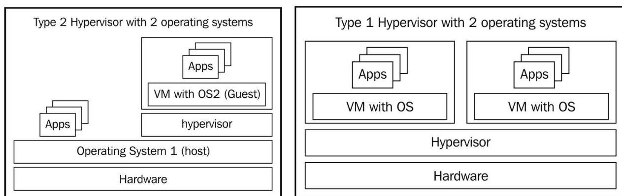
Рис. 1. Різниця між гіпервізором 1 та 2 типу
