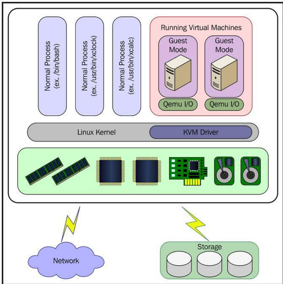
Рис. 3. Візуалізація взаємозв'язків між KVM та QEMU
