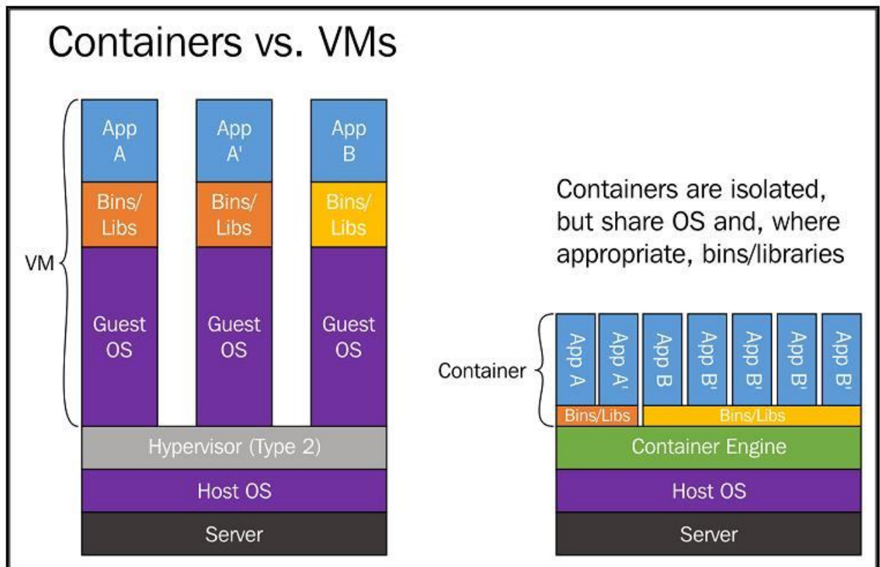
Рис. 4. Порівняння віртуальних машин і контейнерів
